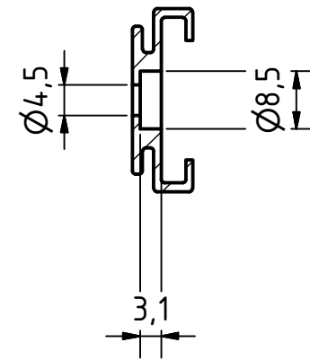
A-A ( 1 : 1 )
