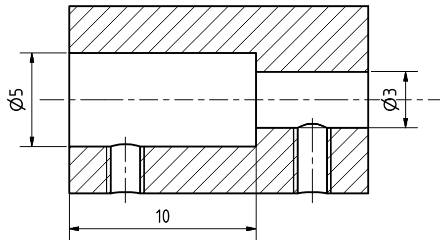
A-A ( 5 : 1 )
